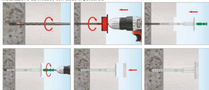
Installazione ad incasso con disco in polistirolo
